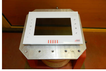
VİBRASYON TESTİ
